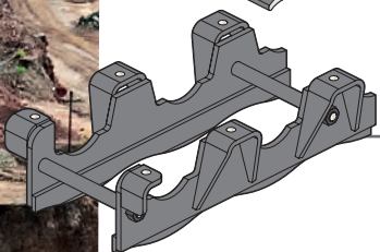
CHAIN GUIDE
